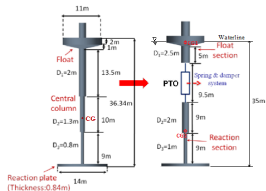
شکل ۱- سیستم مبدهای جاذب نقطه‌ای مبدهای انرژی امواج دریا (مدل لی و همکاران [۲۰])، سمت چپ: سیستم متشکل از یک جسم، راست: سیستم متشکل از دو جسم
