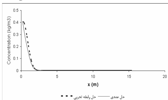
شکل ۱۰ - نمودار تغییرات غلظت در مکان (۵ و x) در T=2.5 s [مبدا مختصات بر روی نقطه رها شده لکه نفتی قرار دارد]
