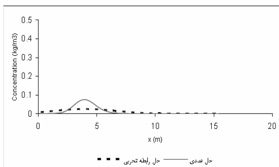
شکل ۱۲ - نمودار تغییرات غلظت در مکان (۵ و x) در T=40 s
