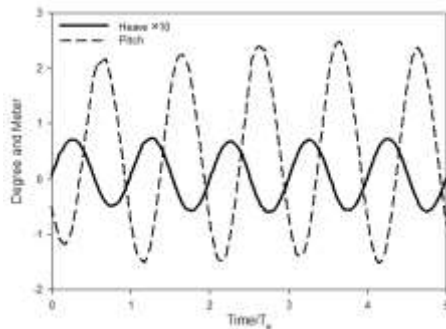
شکل ۱۴- حرکات هیو و پیچ کشتی KCS
