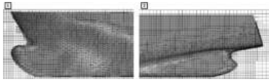
شکل ۷- مش بدنه‌ی کشتی، ۱. سینه کشتی، ۲. پاشنه کشتی
