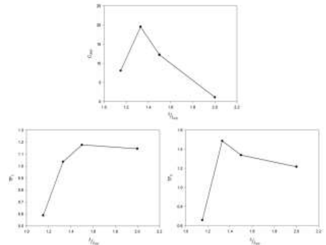
شکل ۲۶- مقایسه‌ی نموداری نتایج شبیه‌سازی مدل کشتی ایران بوشهر در امواج بر حسب نسبت \frac{\lambda}{L_{PP}}
