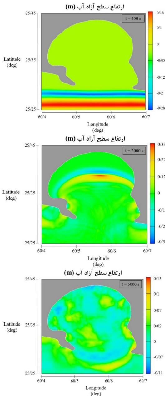
شکل ۴- نتایج شبیه‌سازی انتشار موج سونامی ناشی از گسل مکران در خلیج چابهار در نرم‌افزار Flow 3D
