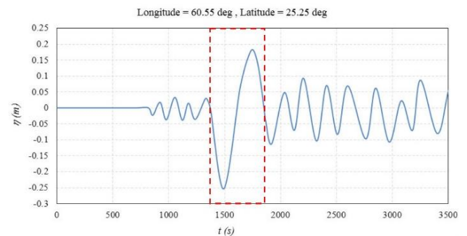
شکل ۳- تغییرات سطح آزاد آب در طول زمان در ابتدای خلیج چابهار مستخرج از مدل سراسری
