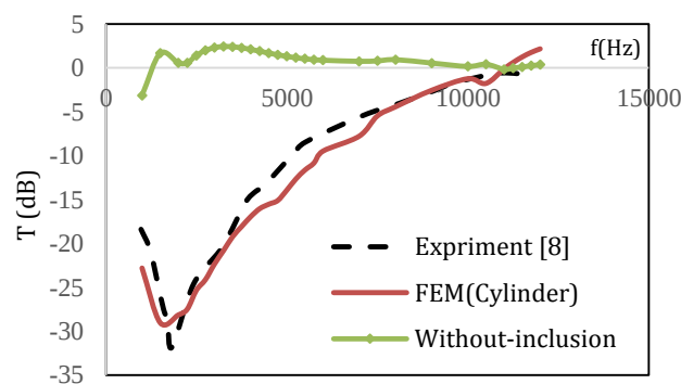
شکل ۹- مقایسه ضریب انتقال برای مدل المان محدود حفره‌دار و بدون حفره وابسته به شبکه
