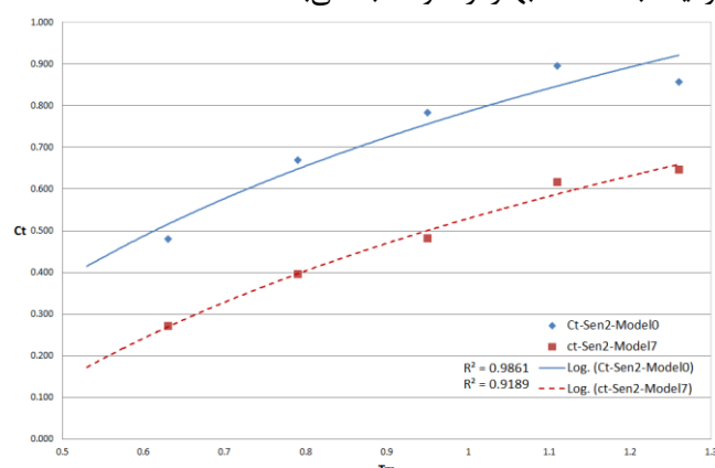
شکل ۱۳: مقایسه عملکرد موج شکن پله ای و مدل مبنا در شبیه سازی گروه دوم
