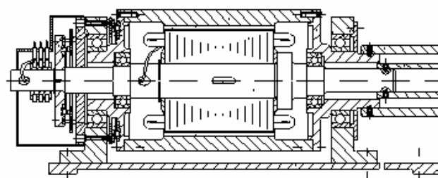
شکل ۲ - مقطع عرضی ساختار معکوس‌گرد [۲۴]
