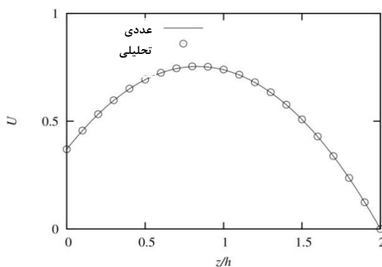
شکل ۲- نمایه سرعت جریان آرام برای حالت Tr=5 به عنوان تابع فاصله از دیوار بدست آمده از حل تحلیلی معادله (۲۴) و عددی
