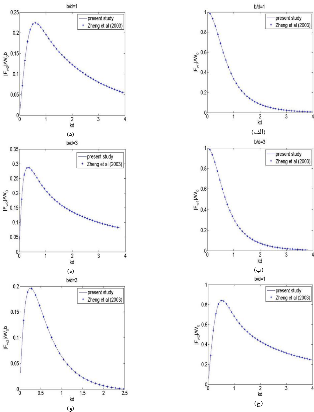
شکل ۴- نیرو و ممان حاصل از موج برای موج شکن دو بعدی با مقطع مستطیلی ( \frac{h}{d} = 2, \frac{b}{d} = 1, 3 )
