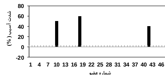
شکل ۹- نتیجه تشخیص آسیب بر اساس روش کاهش گویان با ۴۸ درجه آزادی: (آ) بدون تکرار (ب) با تکرار
