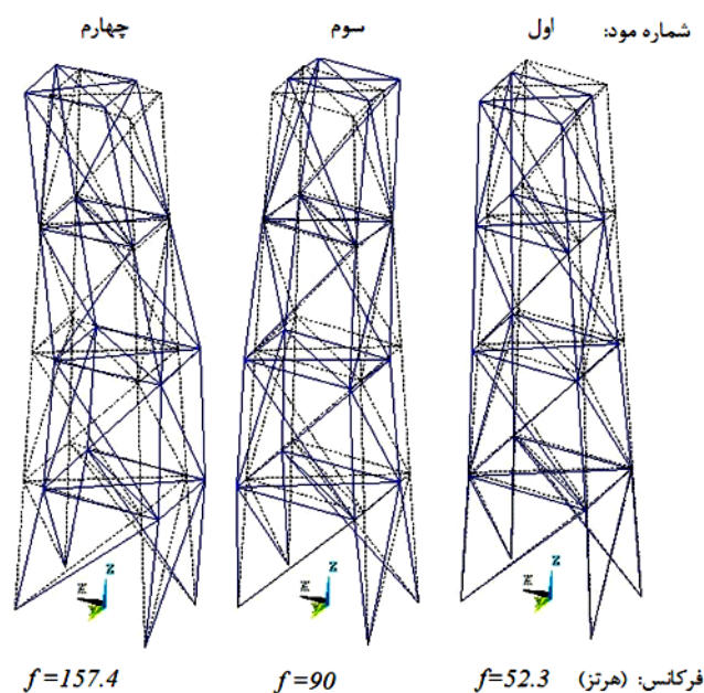
شکل ۴- شکل موده‌های حاصل از تحلیل مودال عددی
