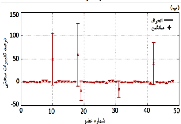
شکل ۱۲- دیاگرام میانگین و انحراف معیار برای نتایج تشخیص عیب با روش مدل کاهش گویان برای دو مقدار مختلف ضریب خطا : \gamma = 1\% (ب) و \gamma = 2\% (آ)
