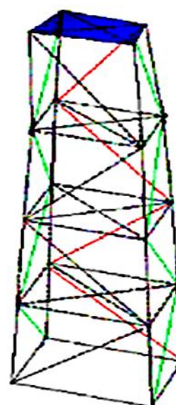
شکل ۵- تحلیل مودال تجربی به همراه شکل مود اول
