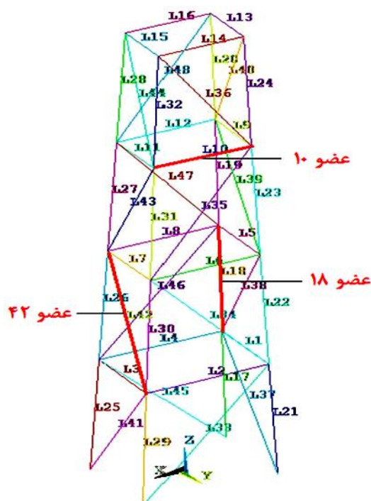
شکل ۸- مدل نهایی المان محدود با ۴۸ عضو
