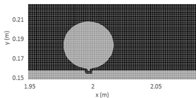
شکل ۳۴- شبکه بندی مورد استفاده در نزدیکی لوله
