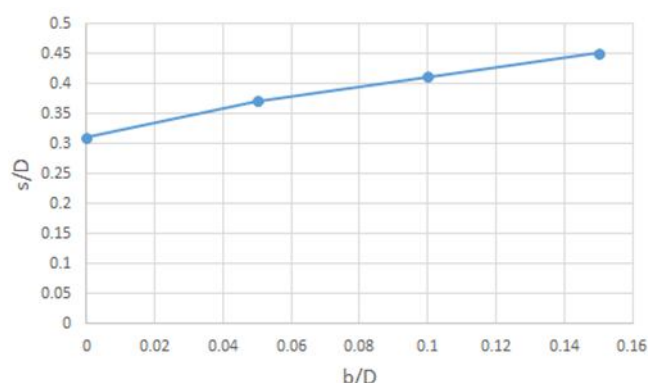
شکل ۹- تغییرات عمق نسبی آبشستگی در مقابل عرض نسبی تیغه برای لوله با قطر ۳/۱ سانتی متر
