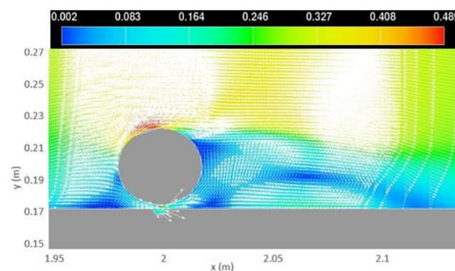
شکل ۳۵- بردارهای سرعت در نزدیکی لوله در زمان ۱۰ ثانیه
