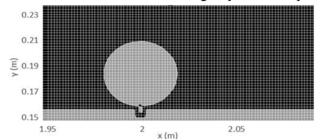
شکل ۳۷- شبکه‌بندی مورد استفاده در نزدیکی لوله
