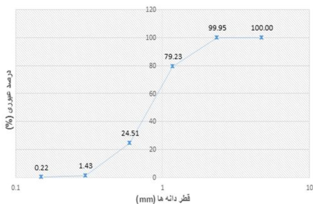
شکل ۳- نمودار دانه‌بندی مصلح بستر
