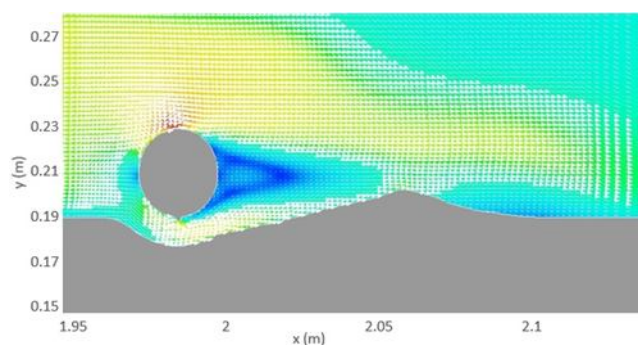
شکل ۳۶- شکل نهائی پروفیل آبشستگی و بردارهای سرعت در زمان ۳۶۰۰ ثانیه
