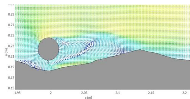
شکل ۳۹- پروفیل نهائی آبشستگی در زمان ۳۶۰۰ ثانیه
