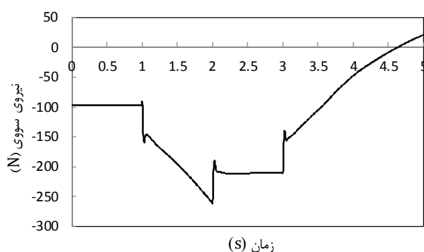
شکل ۱۷- نمودار تغییرات نیروی سووی در حرکت شتابدار سووی
