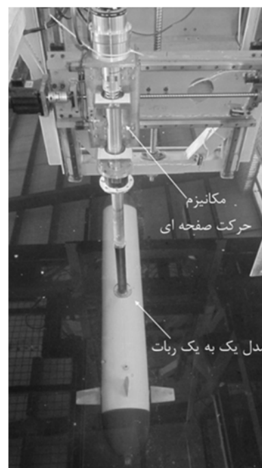
شکل ۱۸- تصویری از مکانیزم حرکت صفحه ای و مدل یک به یک ربات جهت انجام تست های دینامیکی
