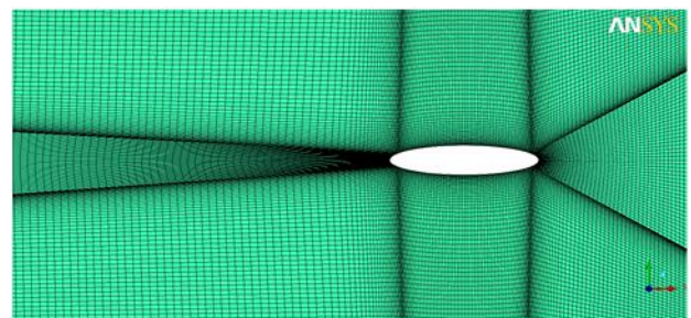
شکل ۷- شبکه با سازمان پیرامون جسم بیضیگون جهت تحلیل حرکت شتابدار در راستای طولی
