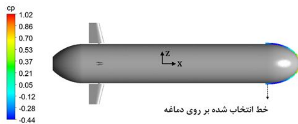
شکل ۱۴- موقعیت خط انتخاب شده بر روی دماغه جهت ترسیم منحنی توزیع ضریب فشار
