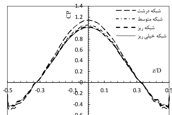
شکل ۱۵- توزیع ضریب فشار بر روی دماغه نسبت به پارامتر بدون بعد z/D برای چهار شبکه مختلف
