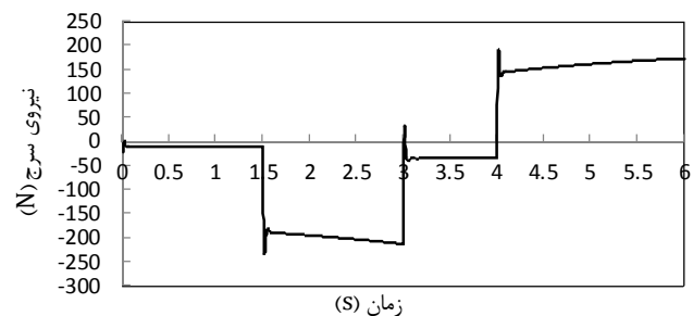
شکل ۸- نمودار تغییرات نیروی وارد بر بیضیگون در راستای طولی در حرکت شتابدار با شتاب ۱ متر بر مجذور ثانیه
