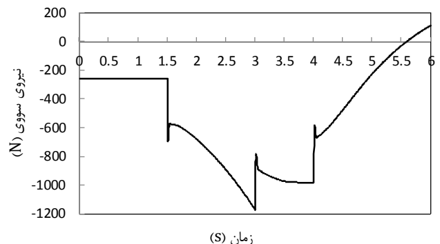
شکل ۹- نمودار تغییرات نیروی وارد بر بیضیگون در راستای عرضی در حرکت شتابدار با شتاب ۱ متر بر مجذور ثانیه
