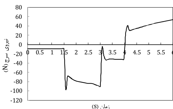
شکل ۱۶- نمودار تغییرات نیروی سرج در حرکت شتابدار سرج
