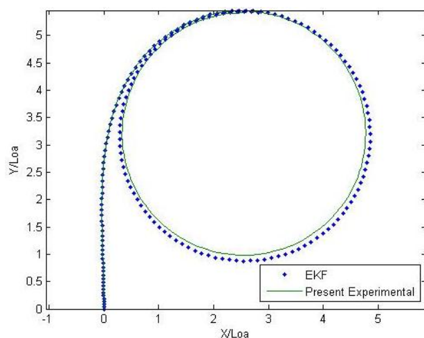
شکل ۹: مقایسه دایره چرخش بدست آمده از تست تجربی و روش شناسایی سیستم
