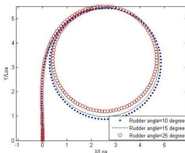
شکل ۱۰: تاثیر زاویه سکان بر دایره چرخش شناور
