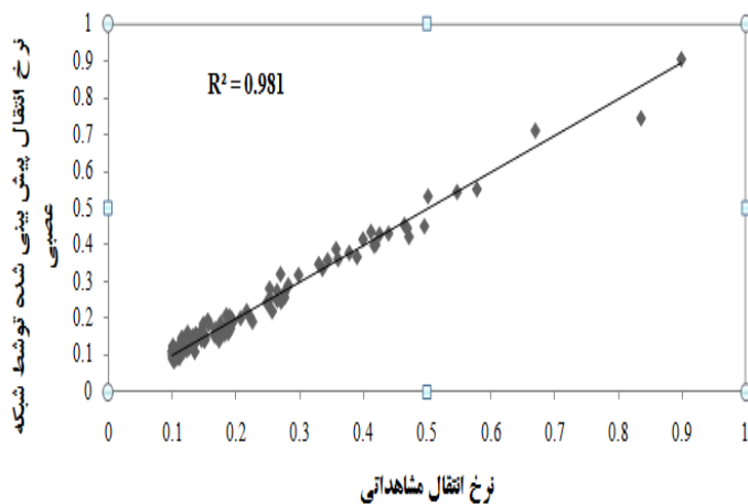
شکل ۵- نمودار پراکندگی نرخ انتقال رسوب پیش بینی شده توسط مدل شبکه عصبی مصنوعی (۵-۱۵).
