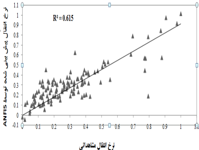
شکل ۶- نمودار پراکندگی نرخ انتقال رسوب در امتداد ساحل پیش بینی شده با استفاده از مدل (MF2)ANFIS
