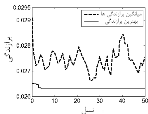
شکل ۶- روند پیشرفت برازندگی کروموزوم‌ها در یک ورق چهار لایه متقارن با ابعاد 1 \times 0.5 m
