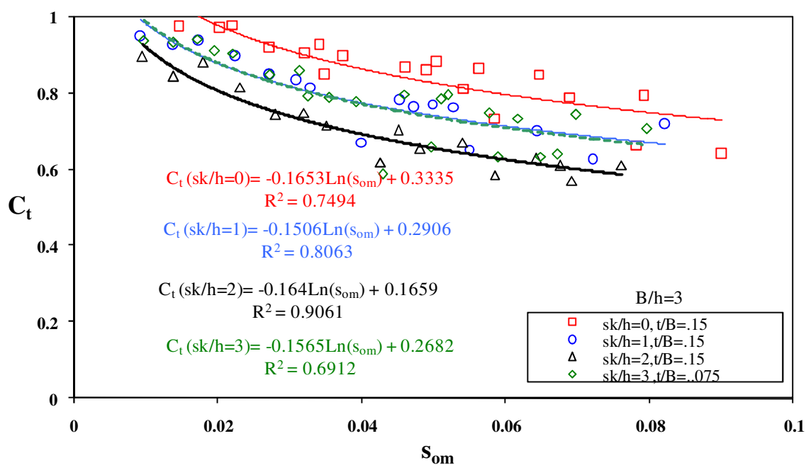
شکل ۹- تغییرات ضرایب انتقال موج برحسب تیزی موج برای موج شکن پانتونی تیغه‌دار با تفکیک نسبت ارتفاع صندوقه به ارتفاع سازه
