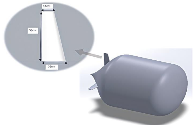
شکل ۱- مدل هندسی زیردریایی تحقیقاتی کوچک مورد استفاده در شبیه‌سازی‌های عددی
