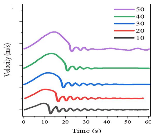
شکل ۲- تغییرات سرعت عمودی زیردریایی در طول فرآیند صعود اضطراری (متر بر ثانیه)
