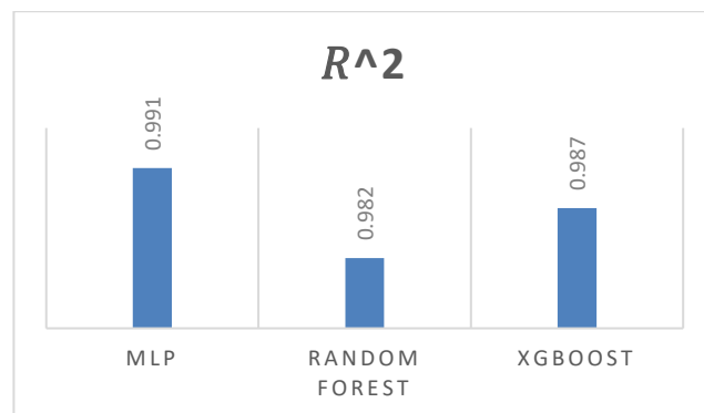
شکل ۳- مقایسه ضریب تعیین مدل‌های یادگیری ماشین
