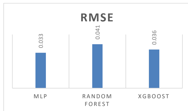
شکل ۴- مقایسه ریشه میانگین مربعات خطای مدل‌های یادگیری ماشین
