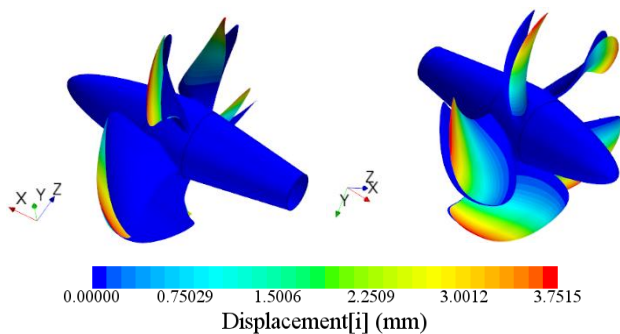
شکل ۳۵: کانتور جابه‌جایی x در J=1.2 و E=0.7 GPa و \nu = 0.33
