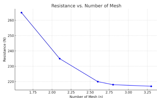
شکل ۸- مقایسه مقاومت شناور ناجی در مش‌بندی‌های مختلف
