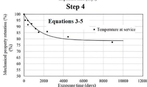
شکل ۲- مدل‌های پیش‌بینی عملکرد بلندمدت با استفاده از تست‌های پیرشدگی تسریع‌شده با استفاده از مدل‌های آرنیوس [۱۳]
