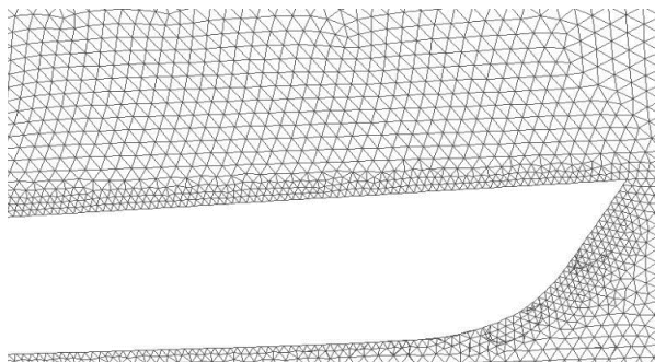
ب) شبکه‌بندی غیرساختاریافته در ناحیه نزدیک بدنه شناور
