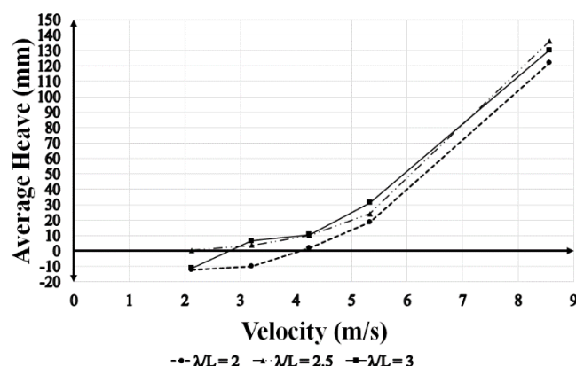
شکل ۱۱- تغییرات متوسط حرکت هيو با سرعت شناور در ۳ نسبت طول موج
