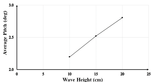
شکل ۱۶- متوسط حرکت پیچ با تغییرات ارتفاع موج در سرعت 5/23 متر بر ثانیه در \lambda/L = 2
