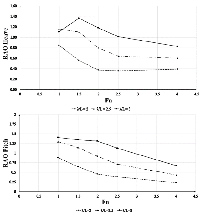
شکل ۱۷- تغییرات عملگر پاسخ دامنه حرکت هیو و پیچ بر حسب فرود حجمی در سه نسبت \lambda/L
