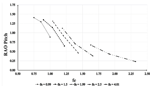
شکل ۱۹-مقادیر عملگر پاسخ دامنه حرکت هیو و پیچ بر حسب فرکانس برخورد در اعداد فرود حجمی مختلف
