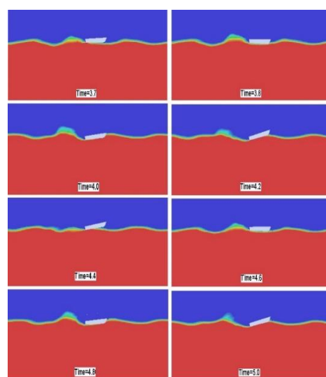
شکل ۸- نمونه‌ای از حرکت شناور در موج در زمانهای مختلف
