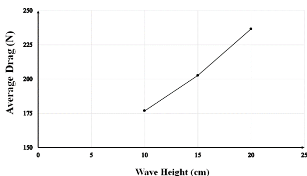
شکل ۱۴- متوسط نیروی پسا با تغییرات ارتفاع موج در سرعت ۵/۲۳ متر
