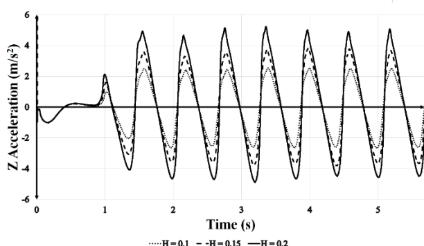
شکل ۱۳-تاریخچه پارامترهای مختلف شناور در سرعت ۵/۲۳ متر بر ثانیه در نسبت ارتفاع های مختلف موج
