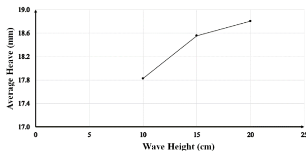
شکل ۱۵- متوسط حرکت هیو با تغییرات ارتفاع موج در سرعت 5/23 متر بر ثانیه در \lambda/L = 2
