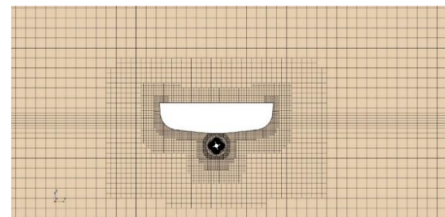
شکل ۱۹ - جزئیات شبکه بندی اطراف لنج و پروانه در صفحات مختلف
