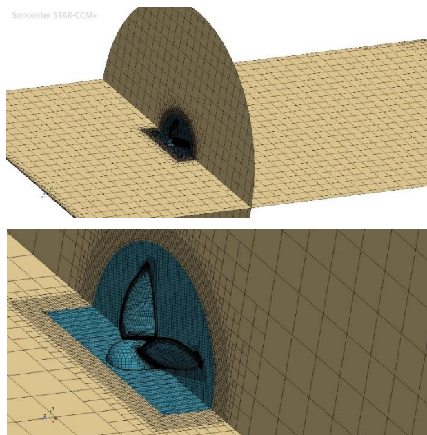
شکل ۱۵- شبکه بندی دامنه حل اطراف پروانه
