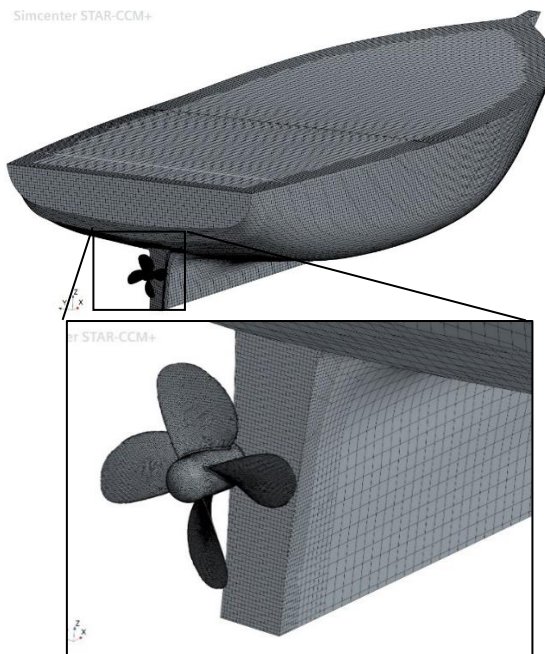
شکل ۱۸- شبکه بندی اطراف لنج و پروانه جهت تست خودرانش
