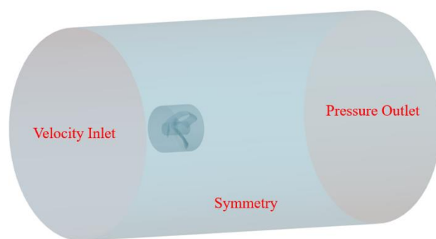
شکل ۱۶- شرایط مرزی دامنه
