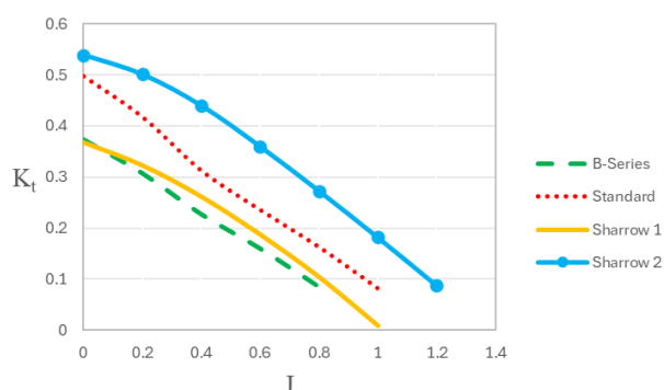
شکل ۳۰- مقایسه ضریب تراست پروانه ها قطر ۰/۴۶۶ متر
