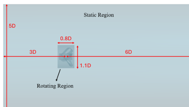
شکل ۱۵- نمایی از دامنه محاسباتی و ابعاد آن
