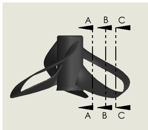
شکل ۷- برش هایی از پره پروانه Sharrow 1
