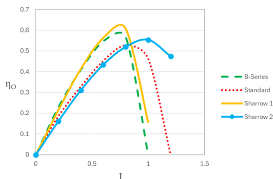
شکل ۳۲- مقایسه بازدهی آب آزاد پروانه ها قطر ۰/۴۶۶ متر
