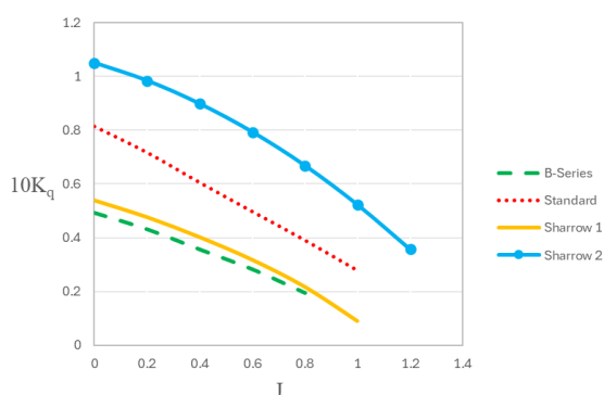
شکل ۳۱- مقایسه ضریب گشتاور پروانه ها قطر ۰/۴۶۶ متر
