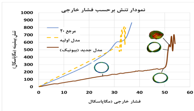
شکل ۱۷ تغییرات تنش ون مایرز نسبت به فشار خارجی
