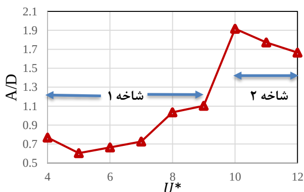
شکل ۸- دامنه بدون بعد استوانه برای سیستم با \gamma = 0.3
