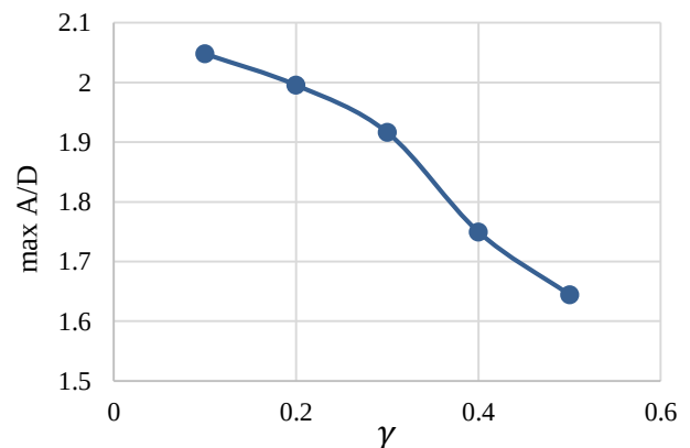
شکل ۲۱- تأثیر مقدار \gamma بر بیشترین دامنه بدون بعد استوانه
