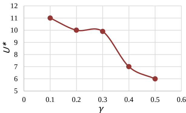
شکل ۲۳- تأثیر مقدار \gamma بر نقطه شروع شاخه ۲
