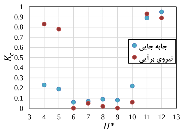
شکل ۱۱- نتایج آزمون ۱-۰ برای سیستم با \gamma = 0.1
