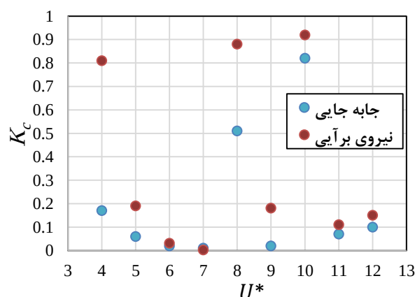
شکل ۱۳- نتایج آزمون ۱-۰ برای سیستم با \gamma = 0.3
