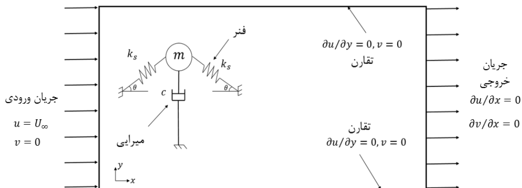
شکل ۱- مدل مورد مطالعه
