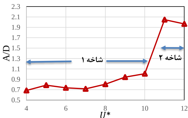
شکل ۶- دامنه بدون بعد استوانه برای سیستم با U^* = 0.1
