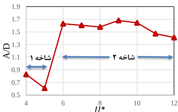
شکل ۱۰- دامنه بدون بعد استوانه برای سیستم با \gamma = 0.5
