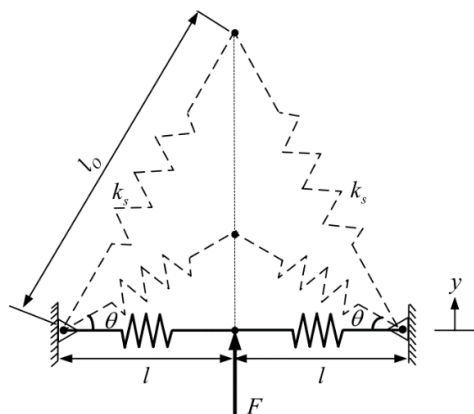
شکل ۲- سیستم ST [۲۵]
