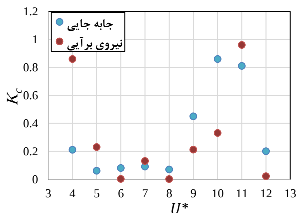
شکل ۱۲- نتایج آزمون ۱-۰ برای سیستم با \gamma = 0.2
