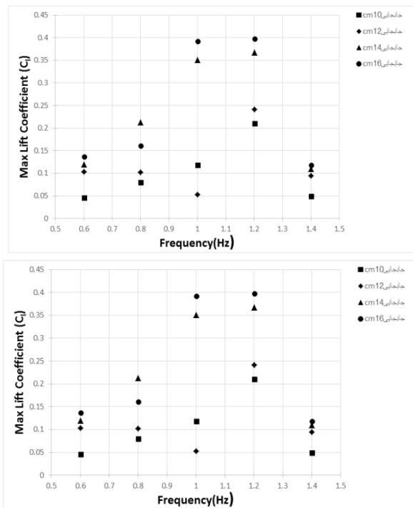
شکل ۱۰- نمودار تغییرات ضریب لیفت ماکزیمم براساس فرکانس‌های مختلف در جابجایی ثابت
