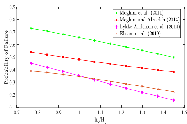
شکل ۱۴- تأثیر پارامتر بدون h_b بر احتمال خرابی سکوی موج‌شکن در مدل‌های مقیم و همکاران (۲۰۱۱)، مقیم و علیزاده (۲۰۱۴)، لیک اندرسن و همکاران (۲۰۱۴) و احسانی و همکاران (۲۰۲۰) در مقطعی با تراز کف ۱۳/۸-
