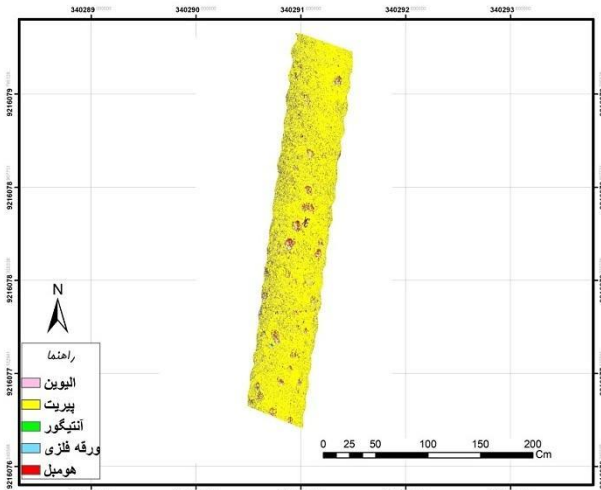
شکل ۴- نقشه بستر اقیانوس با استفاده از الگوریتم نقشه‌برداری زاویه طیفی
