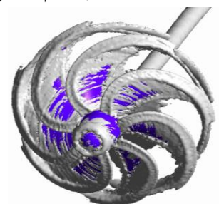
نسبت گام هندسی P/D=1.1
