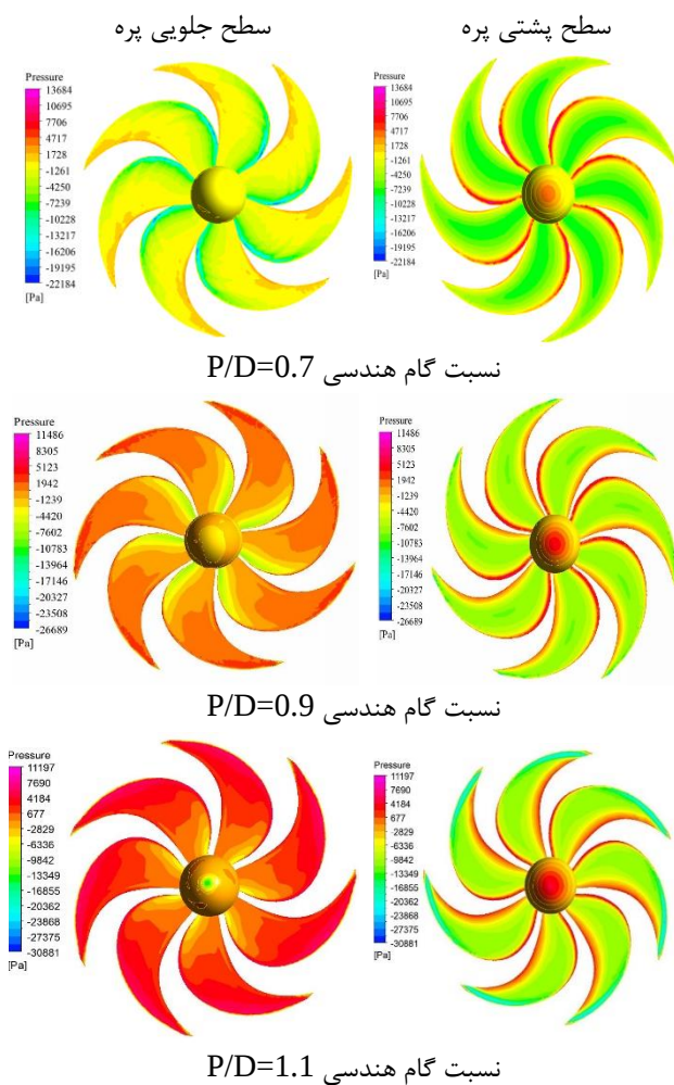
شکل ۱۶- کانتور فشار بر روی سطوح جلویی و پشتی پروانه
