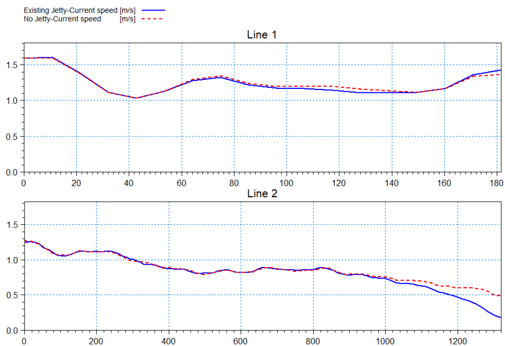
شکل ۱۰- سرعت جریان در امتداد خطوط کنترلی- شرایط دبی ثابت- سیلاب متوسط
