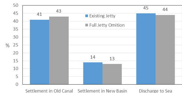
شکل ۲۰- درصد نشست رسوبات در بخش‌های مختلف بندر در
