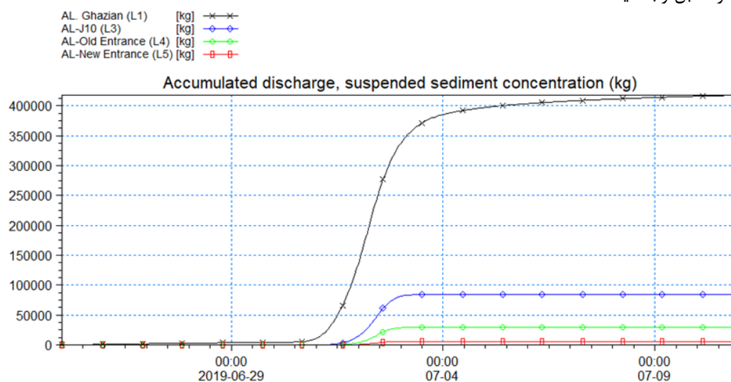
شکل ۱۳-مقادیر تجمعی عبور رسوبات از مقاطع کنترل در سیلاب ضعیف
