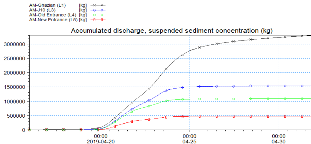
شکل ۱۵-مقادیر تجمعی عبور رسوبات از مقاطع کنترل در سیلاب متوسط- شرایط فعلی اسکله برگشتی
