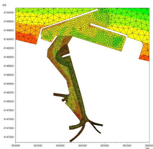
شکل ۶- ابعاد و تراکم متغیر شبکه‌بندی در محدوده شبیه‌سازی
