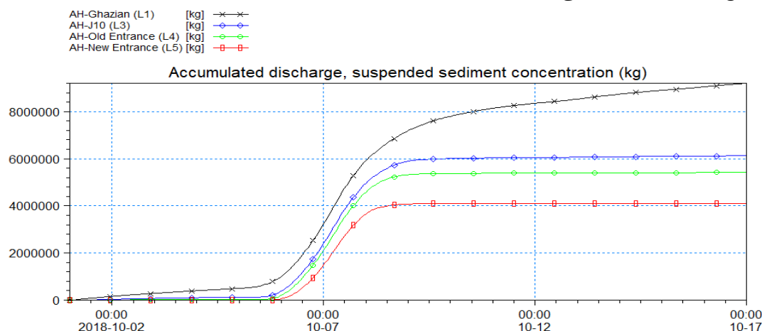
شکل ۱۸- مقادیر تجمعی عبور رسوبات از مقاطع کنترل در سیلاب شدید - شرایط فعلی اسکله برگشتی
