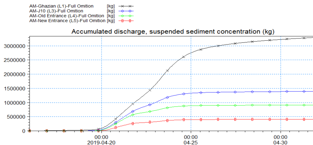
شکل ۱۶-مقادیر تجمعی عبور رسوبات از مقاطع کنترل در سیلاب متوسط- حذف اسکله برگشتی
