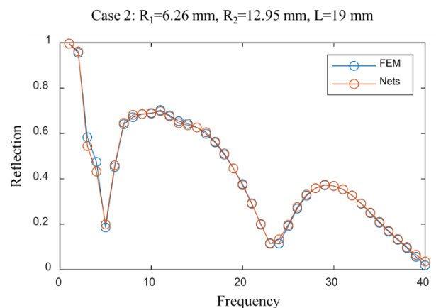
شکل ۱۶: مقایسه پاسخ ضریب انعکاس دو پوشش. خط قرمز پاسخ حاصل از شبکه عصبی و خط آبی پاسخ حاصل از مدل اجزاء محدود
