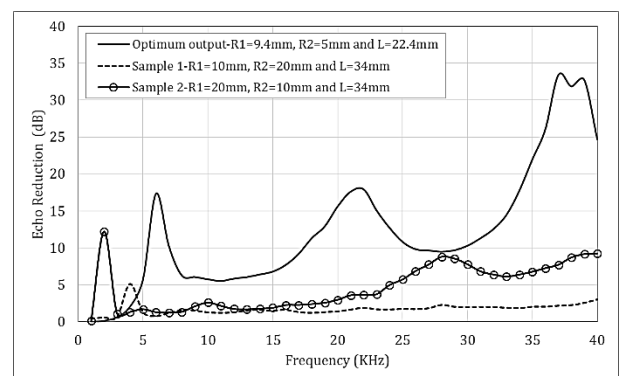
شکل ۲۲: نمودار کاهش اکو برای پاسخ بهینه و دو پاسخ اتفاقی دیگر در بازه‌ی فرکانسی ۱ تا ۴۰ کیلوهرتز
