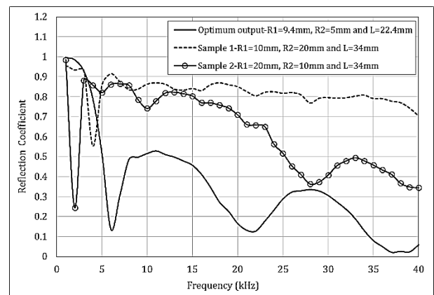
شکل ۲۱: نمودار ضرایب بازتاب برای پاسخ بهینه و دو پاسخ اتفاقی دیگر در بازه‌ی فرکانسی ۱ تا ۴۰ کیلوهرتز
