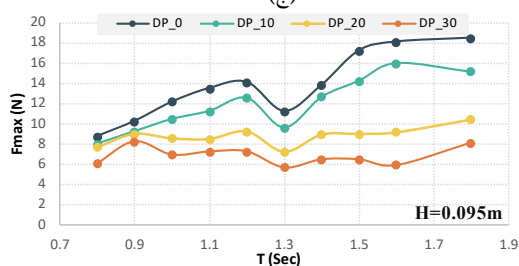
شکل ۴- بیشینه نیرو وارد به مهار جلو سازه های با سطوح مختلف تخلخل بر حسب پریود در ارتفاع امواج مختلف
