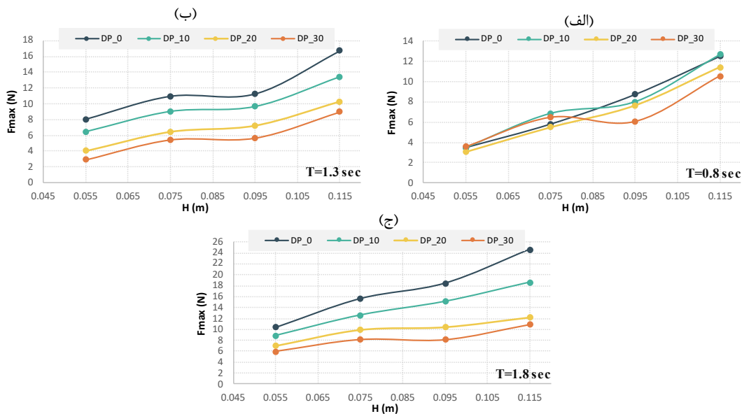
شکل ۶- بیشینه نیرو وارد به مهار جلوسازه‌های با سطوح مختلف تخلخل بر حسب ارتفاع موج در سه نوع پریود (الف) T=0.8 sec: (ب) T=1.3 sec: (ج) T=1.8 sec
