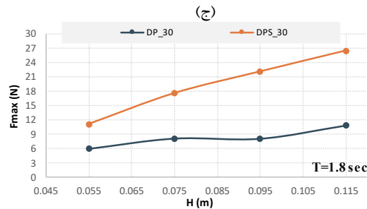
شکل ۹- مقایسه بیشینه نیرو وارد به مهار جلو سازه بین سازه DP_30 و DPS_30 بر حسب ارتفاع موج در سه نوع پرپود موج مختلف T=1.8 sec : (ج) T=1.3 sec : (ب) T=0.8 sec : (الف)
