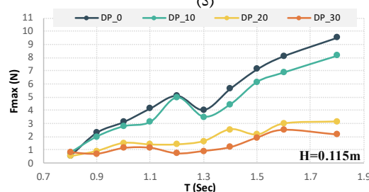
شکل ۵- بیشینه نیرو وارد به مهار پشت سازه های با سطوح مختلف تخلخل بر حسب پریود در ارتفاع امواج مختلف
