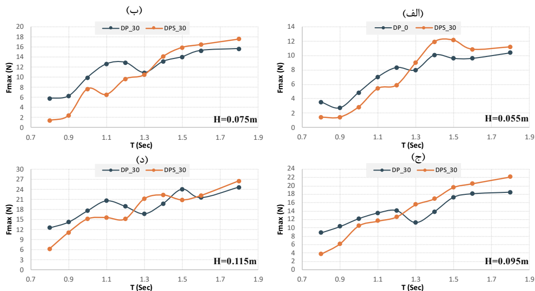
شکل ۷- مقایسه بیشینه نیرو وارد به مهار جلو سازه بین سازه DP_{30} و DPS_{30} بر حسب پریود در ارتفاع امواج مختلف H=0.115m : (د) H=0.095m : (ج) H=0.075m : (ب) H=0.055m : (الف)
