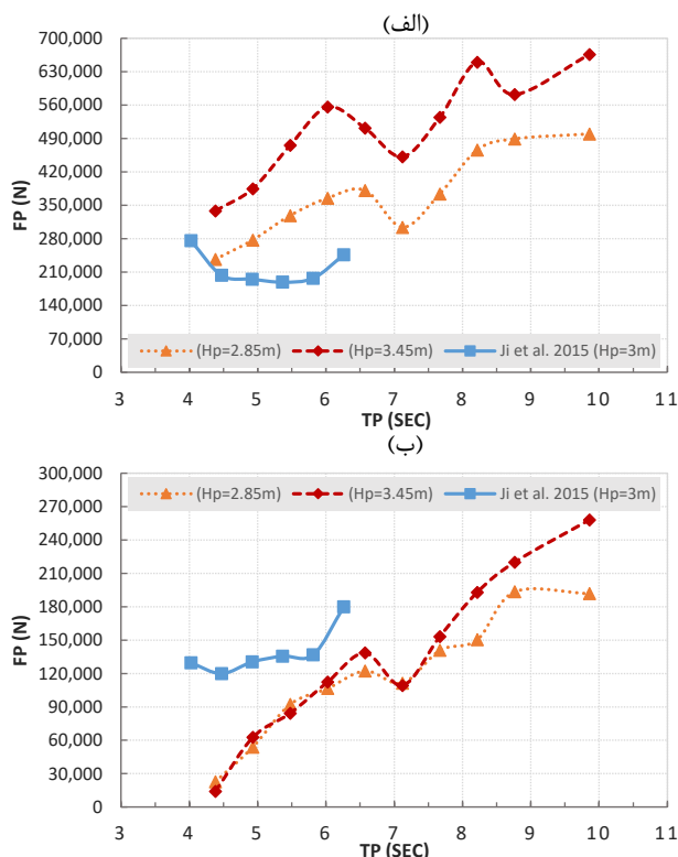
شکل ۱۰- مقایسه بیشینه نیروی مهار جلو و پشت سازه بین پژوهش حاضر و Ji et al. (2015) بر حسب پرپود موج (مقیاس پروتوتایپ): (الف) مهار جلو، (ب) مهار پشت.
