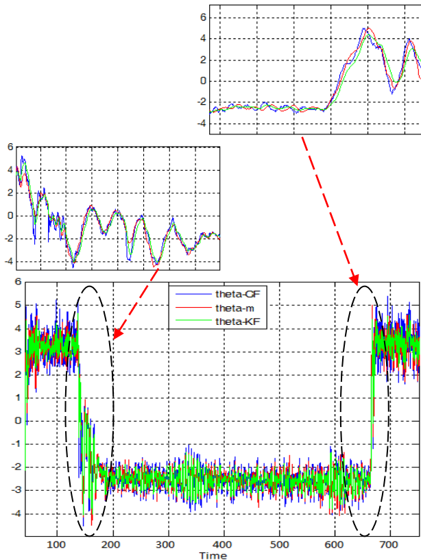
شکل ۷- زاویه فراز اندازه گیری شده و تخمین زاویه فراز با فیلتر CF تطبیقی و کالمن (درجه)
