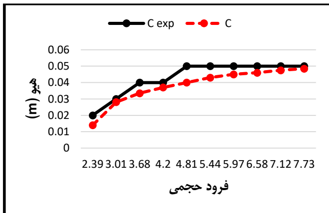
شکل ۱۱- نمودار هیو بر حسب فرود حجمی شناور پروازی C در شبیه‌سازی‌های عددی صورت گرفته و داده‌های آزمایشگاهی
