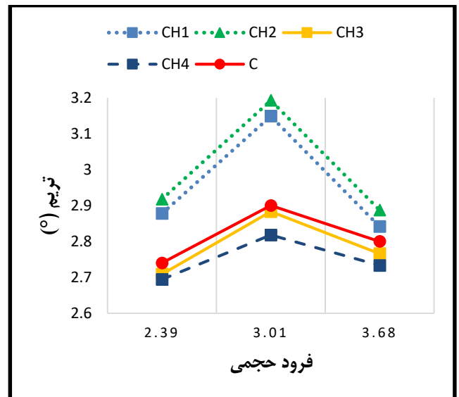
شکل ۲۴- نمودار ترسیم شناورهای پروازی در مقایسه با هم در شبیه سازی های عددی صورت گرفته در فرود حجمی ۲/۳۹، ۳/۰۱ و ۳/۶۸
