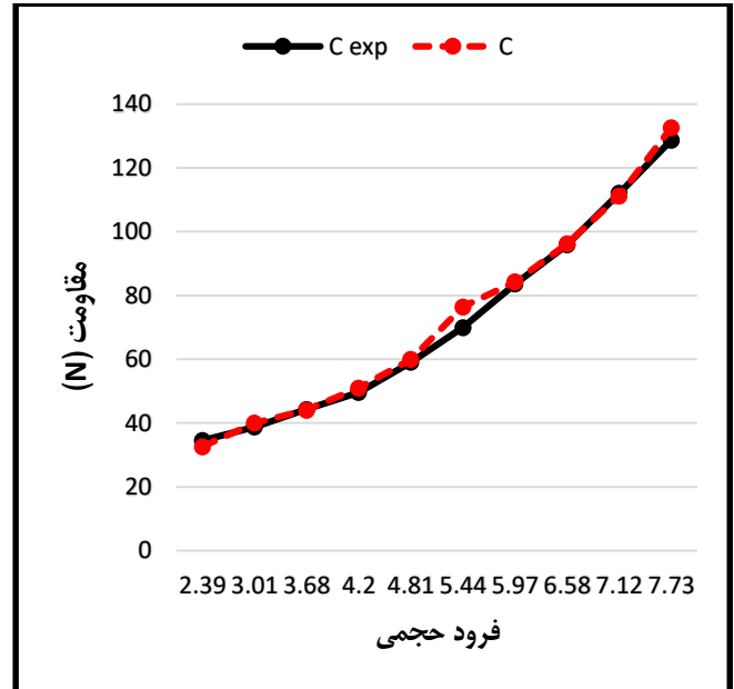
شکل ۹- نمودار مقاومت بر حسب فرود حجمی شناور پروازی C در شبیه‌سازی‌های عددی صورت گرفته و داده‌های آزمایشگاهی
