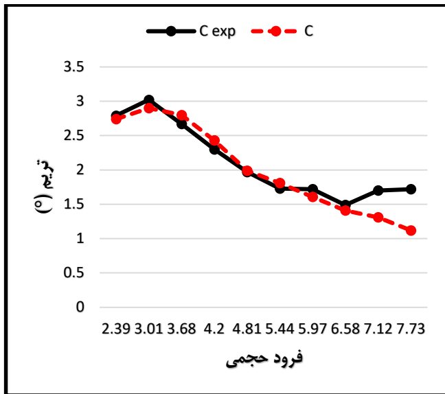
شکل ۱۰- نمودار تریم بر حسب فرود حجمی شناور پروازی C در شبیه‌سازی‌های عددی صورت گرفته و داده‌های آزمایشگاهی
