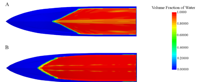
شکل ۱۳- کانتور کسر حجمی سیال سطح خیس شناور پروازی C. A) فرود حجمی ۲/۳۹، B) فرود حجمی ۵/۴۴
