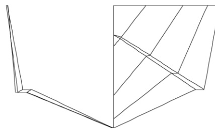
شکل ۲- خطوط بدنه شناور پروازی C از سری ساتهمپتون از نمای روبرو ارائه شده [۸]
