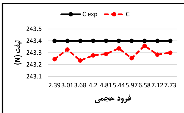
شکل ۱۲- نمودار لیفت بر حسب فرود حجمی شناور پروازی C در شبیه‌سازی‌های عددی صورت گرفته و داده‌های آزمایشگاهی
