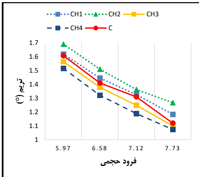
شکل ۲۲- نمودار ترسیم شناورهای پروازی در مقایسه با هم در شبیه سازی های عددی صورت گرفته در فرود حجمی ۵/۹۷، ۶/۵۸، ۷/۱۲ و ۷/۷۳
