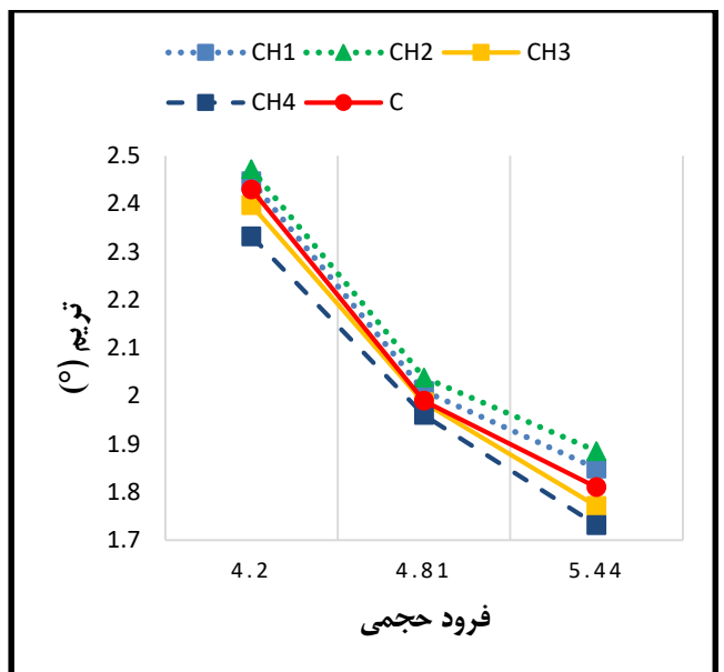
شکل ۲۵- نمودار ترسیم شناورهای پروازی در مقایسه با هم در شبیه سازی های عددی صورت گرفته در فرود حجمی ۴/۲، ۴/۸۱ و ۵/۴۴
