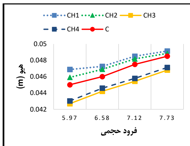
شکل ۲۶- نمودار هیو شناورهای پروازی در مقایسه با هم در شبیه-سازی‌های عددی صورت گرفته در فرود حجمی ۵/۹۷، ۶/۵۸، ۷/۱۲ و ۷/۷۳
