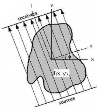
شکل ۱- چشمه-گیرنده‌ی چرخان [۵].
