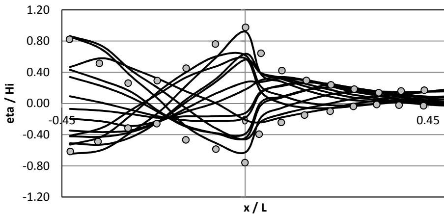
شکل ۶- سری‌های زمانی پروفیل‌های سطحی آب با فواصل زمانی T / 14 در طول یک دوره تناوب. نقاط دایره‌ای، نسبت ترازهای اندازه‌گیری شده اوج و حوض موج ( \eta ) به ارتفاع موج اولیه ( H_i ) در آزمایش هستند.
