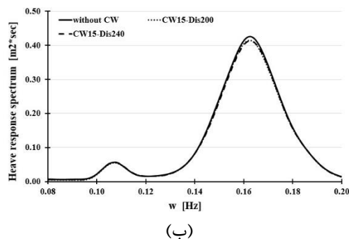
شکل ۱۴- طیف حرکت هیو، الف-محدوده فرکانس پایین، ب- محدوده فرکانس بالا
