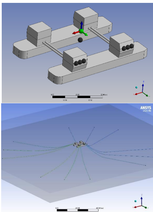
شکل ۳- مدل سکوی نیمه مغروق به همراه خطوط مهار در نرم‌افزار ANSYS
