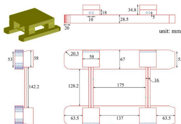
شکل ۲- ابعاد مدل شناور نیمه مغروق با مقیاس ۱:۳۰۰ [۱۹]
