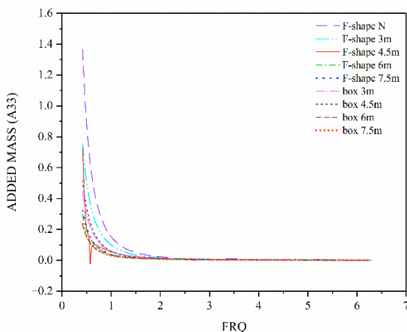
شکل ۹- تغییرات ضریب جرم افزوده در راستای قائم بر حسب فرکانس در اعماق مختلف فرورفت موج شکن
