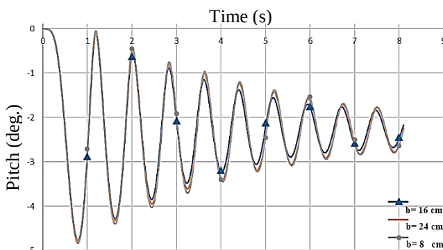
شکل ۱۶- نمودار حرکت پیچ شناور با پایدارساز هیدروفویلی زاویه‌دار با سه عرض میانی مختلف
