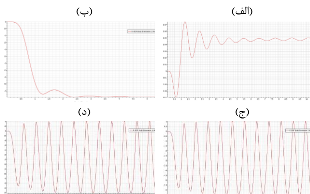
شکل ۱۱ - نمودار حرکت پیچ-زمان شناور در سرعت‌های مختلف
