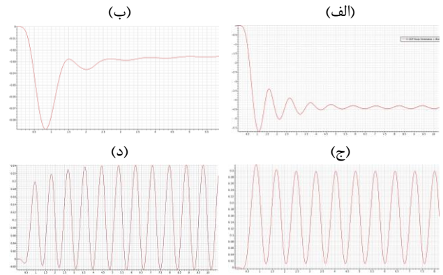
شکل ۱۲- نمودار حرکت هیو-زمان شناور در سرعت‌های مختلف (الف): ۱۵ گره، (ب): ۲۰ گره، (ج): ۳۰ گره، (د): ۴۰ گره [۳۰]
