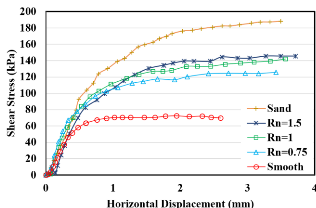
شکل ۹- اثر زبری نسبی سطح فولاد برای ماسه کربناته با دانسیته نسبی ۳۰٪ در تنش نرمال ۲۵۰ کیلوپاسکال
