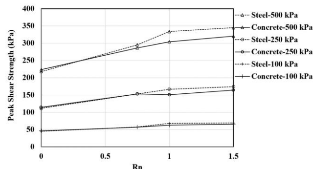
شکل ۱۹- مقادیر مقاومت برشی ماکزیمم برای ماسه کربناته با دانسیته نسبی ۹۰ درصد به ازای زبری متفاوت سطح فولادی و بتنی
