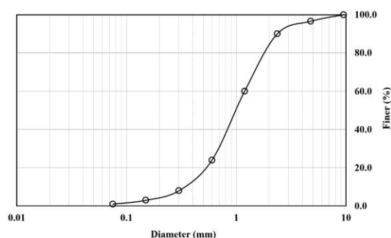
شکل ۳- منحنی دانه‌بندی ماسه کربناته
