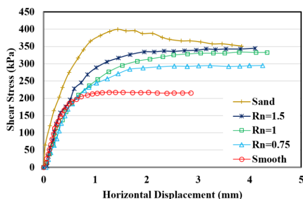
شکل ۱۳- اثر زبری نسبی سطح فولاد برای ماسه کربناته با دانسیته نسبی ۹۰٪ در تنش نرمال ۵۰۰ کیلوپاسکال
