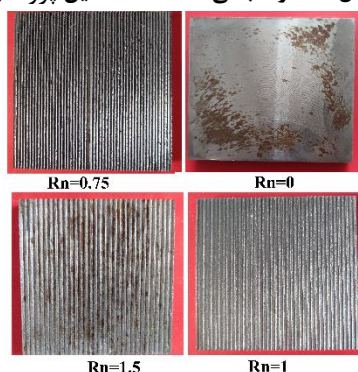
شکل ۵- نمونه فولادی ساخته شده این پژوهش
