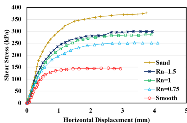
شکل ۱۰- اثر زبری نسبی سطح فولاد برای ماسه کربناته با دانسیته نسبی ۳۰٪ در تنش نرمال ۵۰۰ کیلوپاسکال
