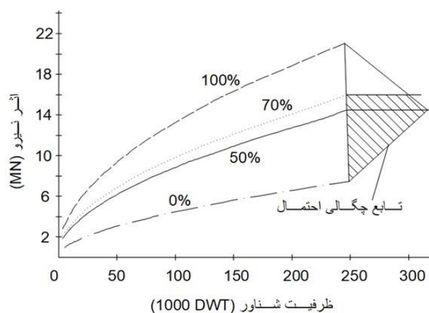
شکل ۴: توزیع احتمال نیروی ناشی از برخورد شناور [۱۲]
