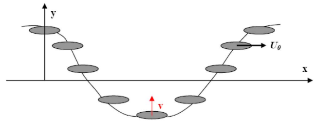
شکل ۳ - وضعیت مانور مدل در تست سوی خالص
