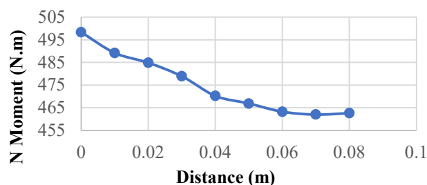
شکل ۹ - نمودار گشتاور یاو بر حسب فاصله سطوح کنترلی از بدنه
