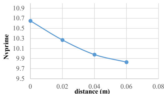
شکل ۱۱ - نمودار ضریب هیدرودینامیکی N_v' بر حسب فاصله سطوح کنترلی از بدنه
