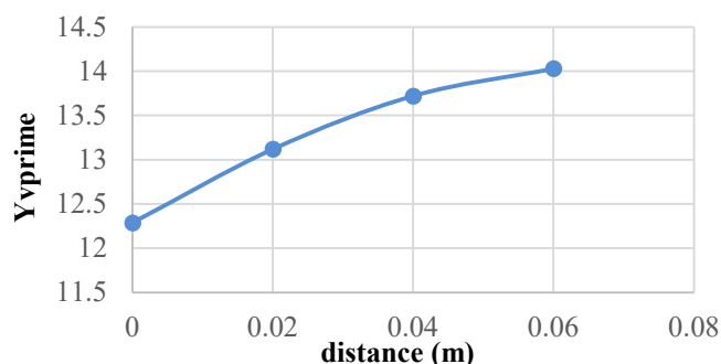
شکل ۱۰ - نمودار ضریب هیدرودینامیکی Y_v' بر حسب فاصله سطوح کنترلی از بدنه
