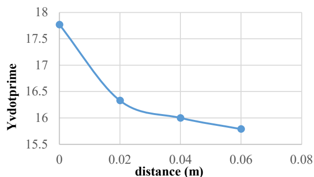
شکل ۱۲ - نمودار ضریب هیدرودینامیکی Y_v' بر حسب فاصله سطوح کنترلی از بدنه
