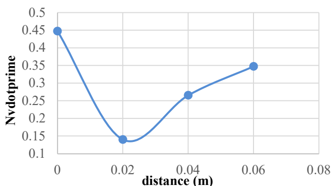
شکل ۱۳ - نمودار ضریب هیدرودینامیکی N_v' بر حسب فاصله سطوح کنترلی از بدنه
