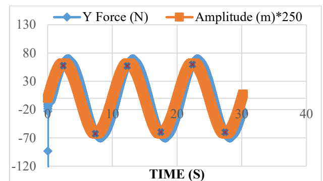
شکل ۴ - نمایش نقاط سرعت صفر برای استخراج نیرو و ممان
