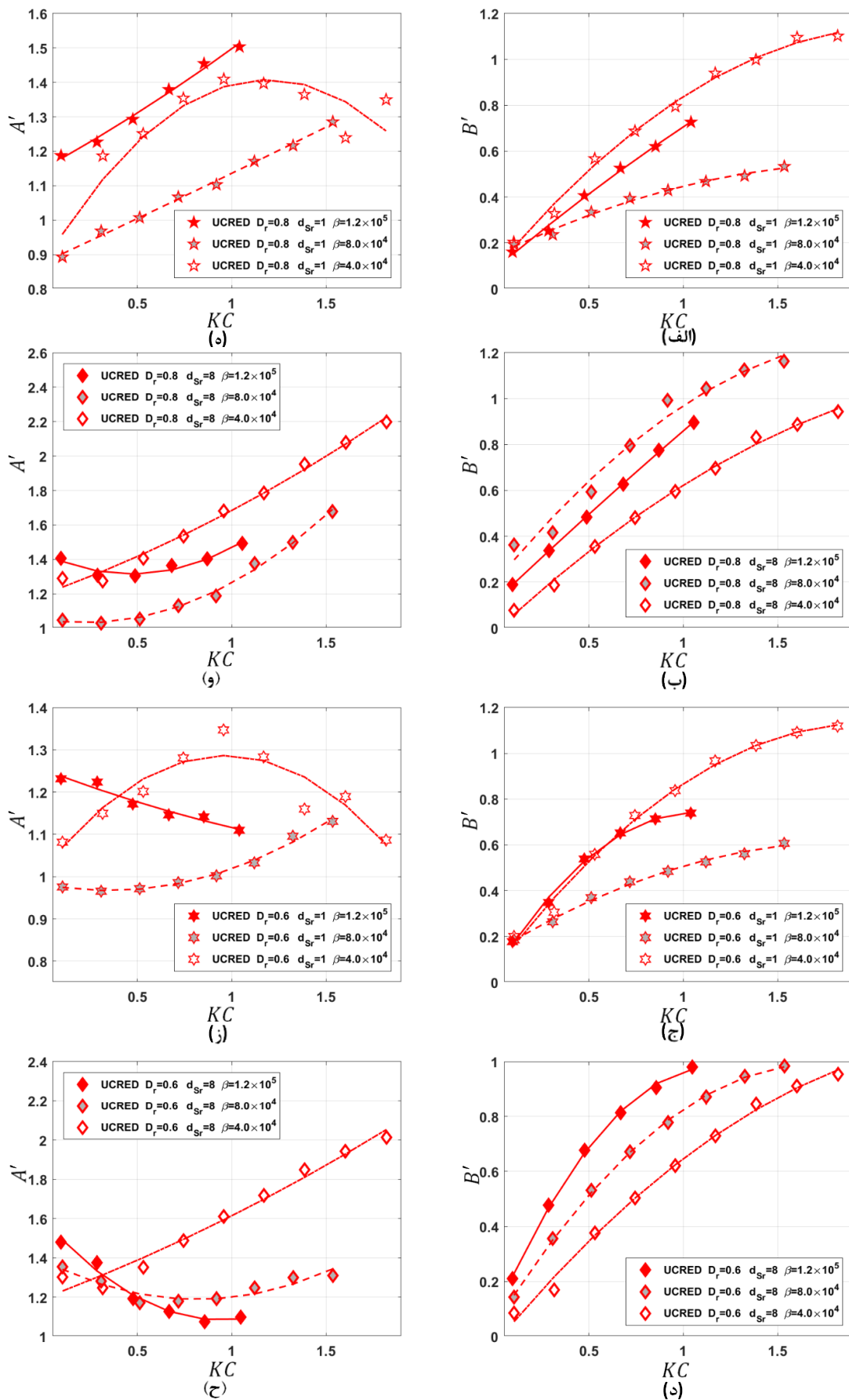
شکل ۹- تأثیر B' روی ضرایب هیدرودینامیک دیسک ترکیبی UCRD با D_r های مختلف در موقعیت نزدیک به سطح و کف.
