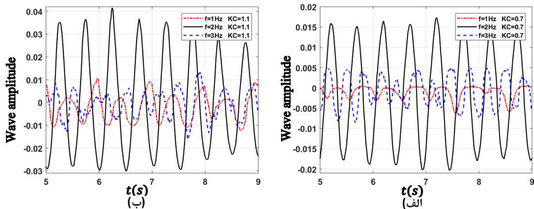
شکل ۶- دامنه امواج تشعشعی سطح آزاد آب برای نمونه FRD با d_{Sr} = 1 . (الف) KC = 0.7 ، (ب) KC = 1.1 .
