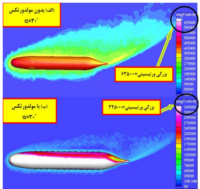
شکل ۴: مقایسه جریان گردابه‌ای و ورتیسیتیته اطراف بدنه زیرسطحی سابوف در زاویه حمله ۳۰ درجه (بدون مولد ورتکس (بالا) و با مولد ورتکس (پایین)).
