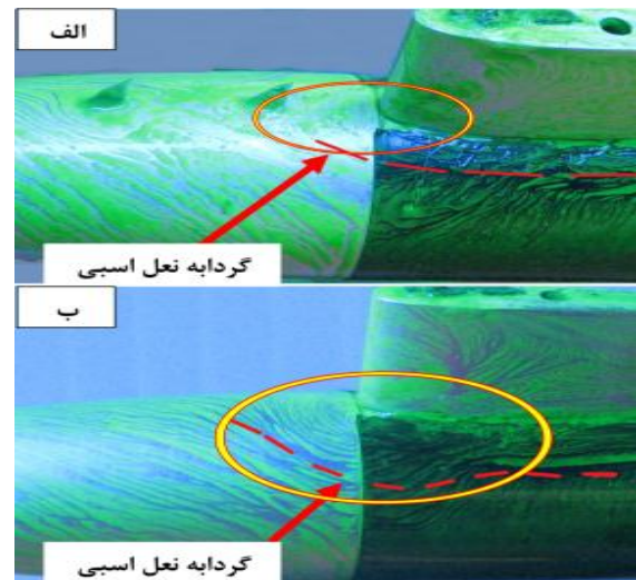
شکل ۱۳: مکان گردابه نعل اسبی جریان بر روی مدل زیرسطحی سابوف برای دو حالت بدنه با مولد ورتکس (در شکل بالا راست و در شکل پایین الف می‌باشد) و بدنه بدون مولد ورتکس (در شکل بالا چپ و در شکل پایین ب می‌باشد) در زاویه حمله ۳۰ درجه.
