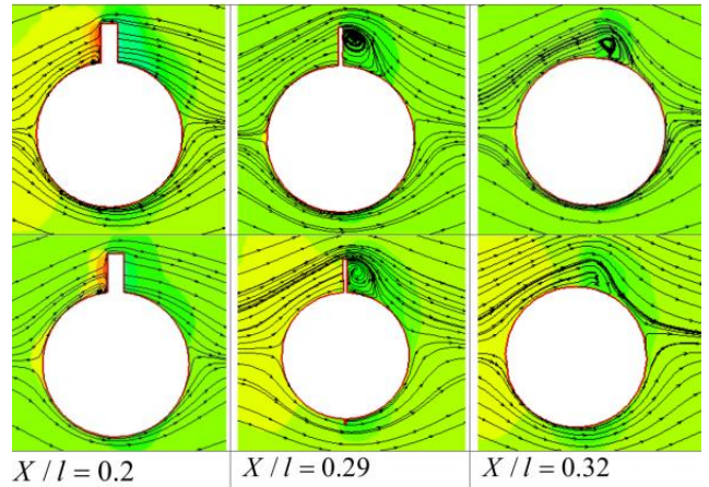
شکل ۱۰: کانتور فشار اطراف مدل در مقاطع مختلف و خطوط جریان در اطراف بدنه زیرسطحی سابوف در مقاطع مختلف در نزدیک محدوده اتصال برجک به بدنه و در زاویه حمله ۳۰ درجه (بدون مولد ورتکس (بالا) و با مولد ورتکس (پایین)).
