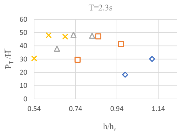
شکل ۱۱ ب: تغییرات بدون بعد فشار خروجی در برابر عمق آب برای دوره تناوب ۲.۳s
