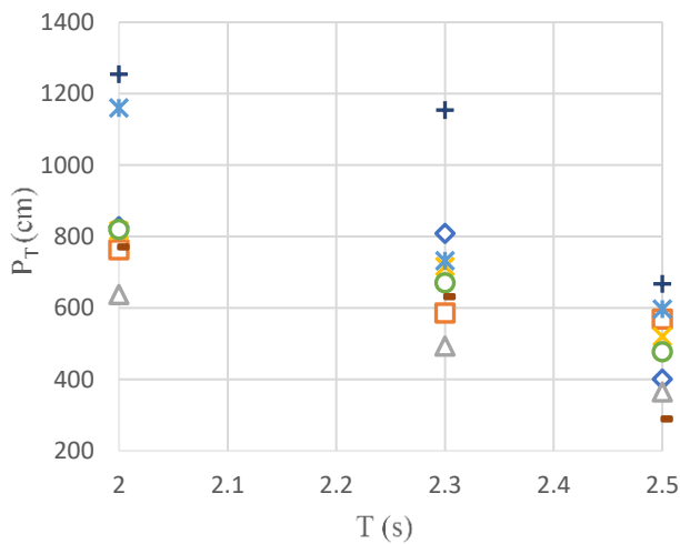
شکل ۱۶: تغییرات فشار خروجی در برابر دوره تناوب موج برای شیب ۱:۳
