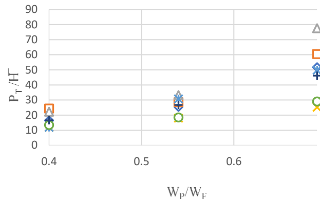
شکل ۹: نمودار بدون بعد تاثیر عرض صفحه دستگاه مبدل انرژی بر فشار تولیدی
