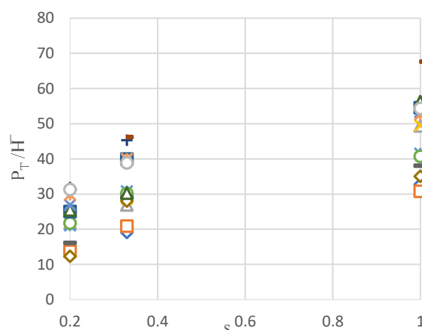
شکل ۱۳: نمودار بدون بعد تأثیر شیب ساحل بر فشار تولیدی
