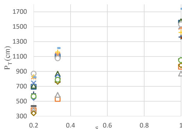
شکل ۱۲: تأثیر شیب ساحل بر فشار تولیدی
