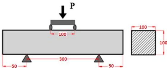
شکل ۴ - آزمایش خمشی ۴ نقطه‌ای
