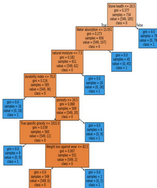
شکل ۱- خروجی الگوریتم درخت تصمیم
