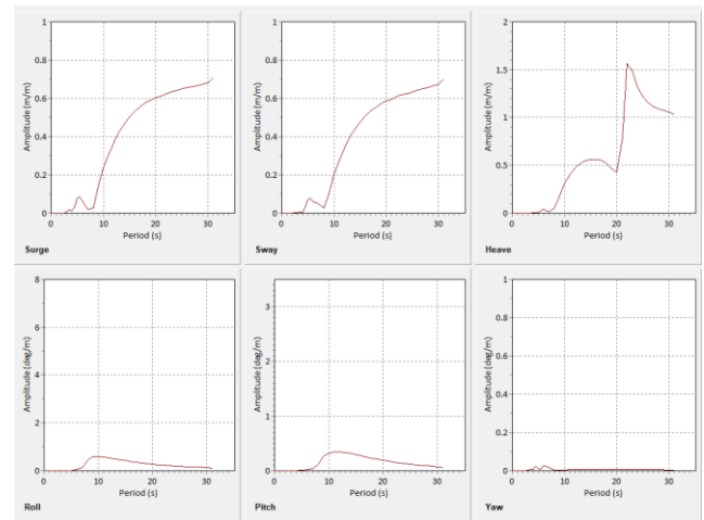
شکل ۱۳- دامنه طیف پاسخ در زاویه ۴۵ درجه
