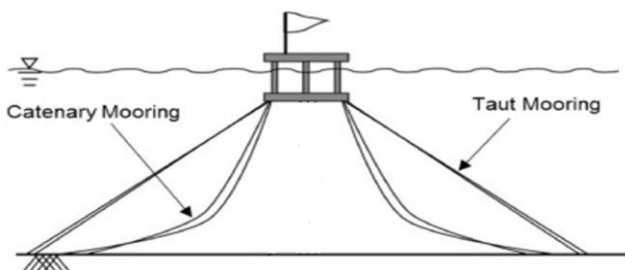
شکل ۲ - انواع سیستم مهار کششی - کنتری [۳]
